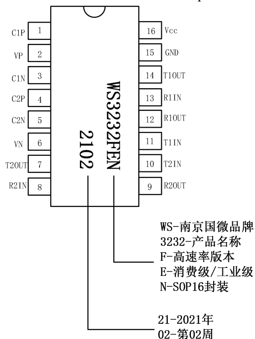
WS3232F 引脚图—16-pin SOP (Top View)
