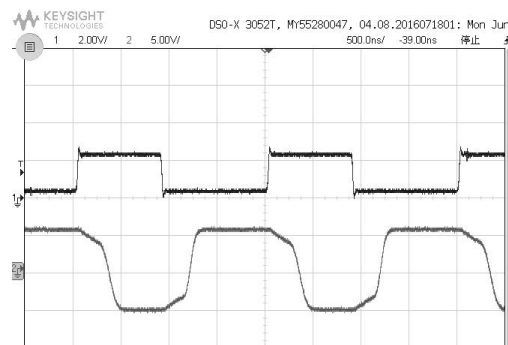
图 1. WS3232F TIN to TOut (3K&amp;250pF load) at 1000kbps waveform
