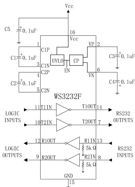
图 6 WS3232F 典型外围应用电路
